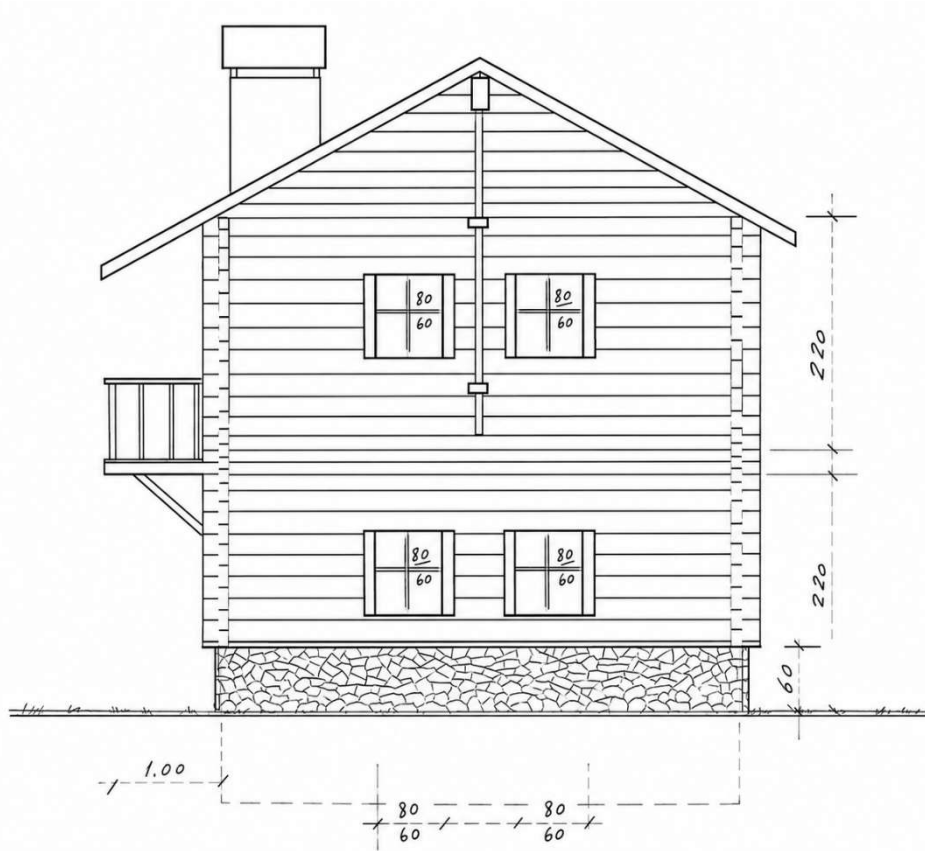
Façade est
