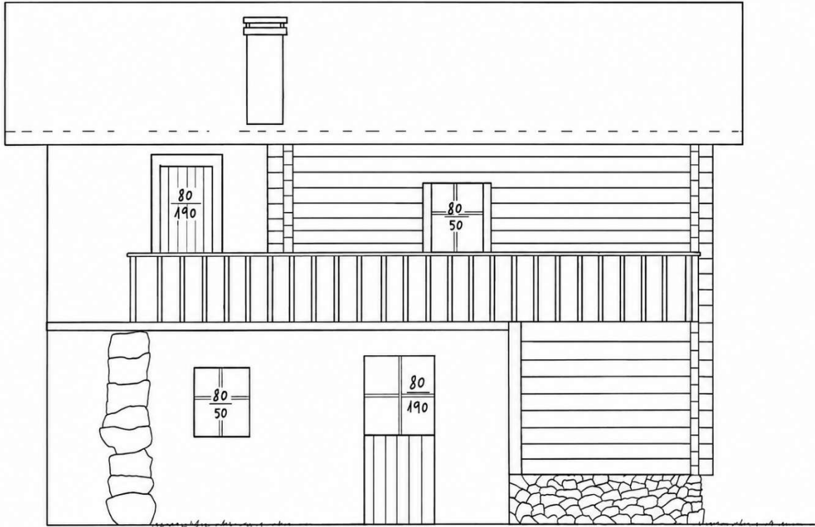
Façade sud
