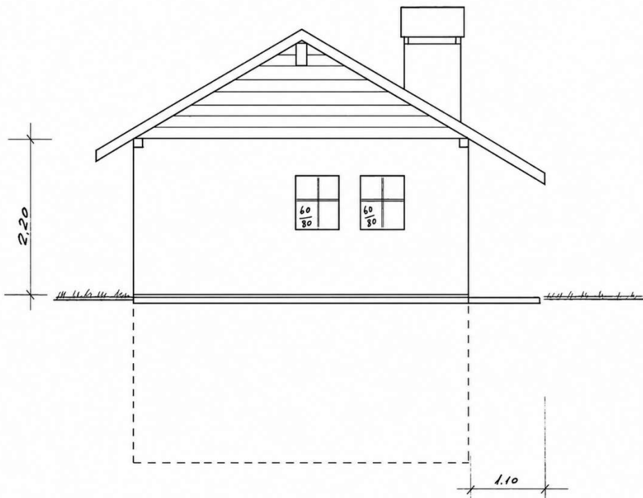
Façade ouest
