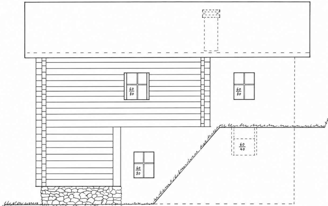
Façade nord
