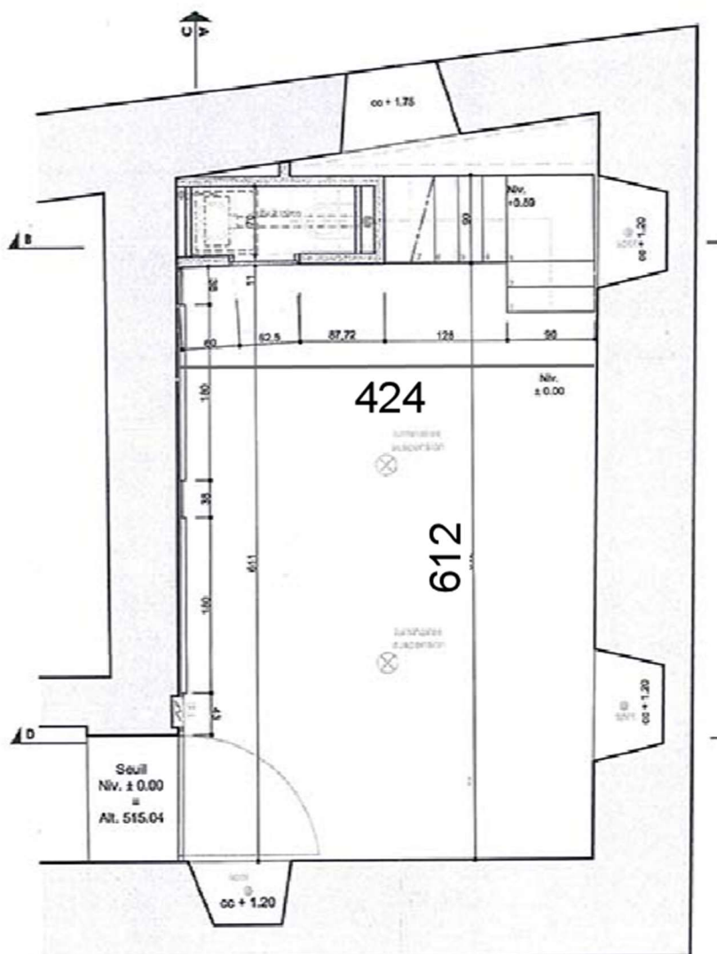
Plan du sous-sol
